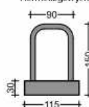
Listwa czwujęciowa Ø 10 mm dla elementów prefabrykowanych i formsiłazowych h
